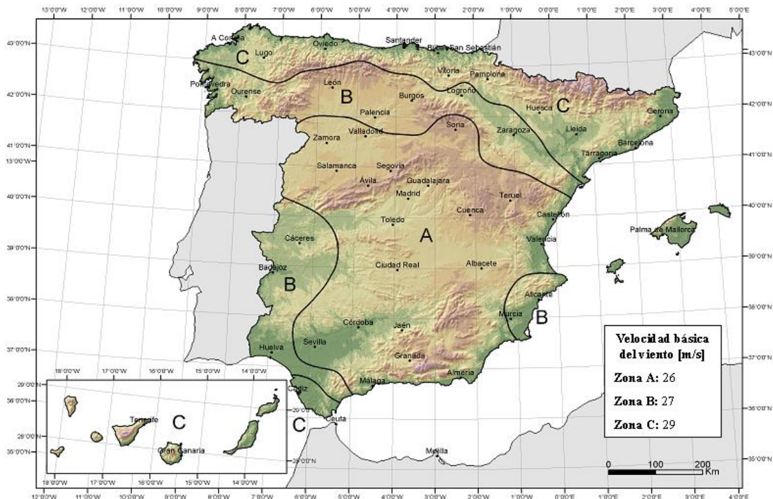
Figura 2.5 Zonas eólicas
